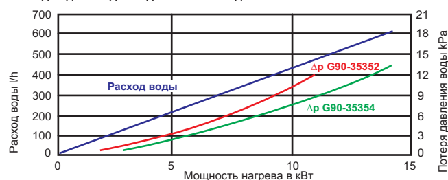
Расход воды и падение давления по воде
