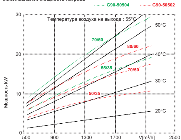
Максимальная мощность нагрева
