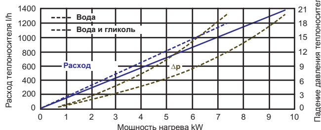
Расход воды и падение давления по теплоносителю
