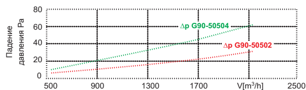
Расход воды и падение давления по воде
